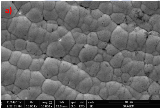
Şekil 1.2. Akımsız Ni-B-P kaplaya ait SEM görüntüsü; a) Yüzey ve b) Kesit görüntüsü
